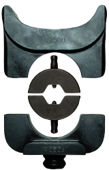
Övre backhållare V2508, B-backar, nedre backhållare V2506
