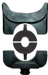
Övre backhållare V2508, BC-backar, nedre backhållare V2506
